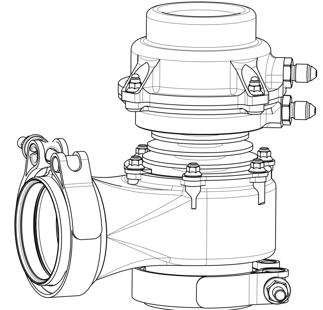
Isometric view Scale: 1:1
